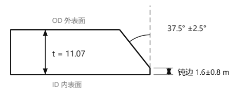
端部坡口详图 · ASME B16.25-2017 · NTS
